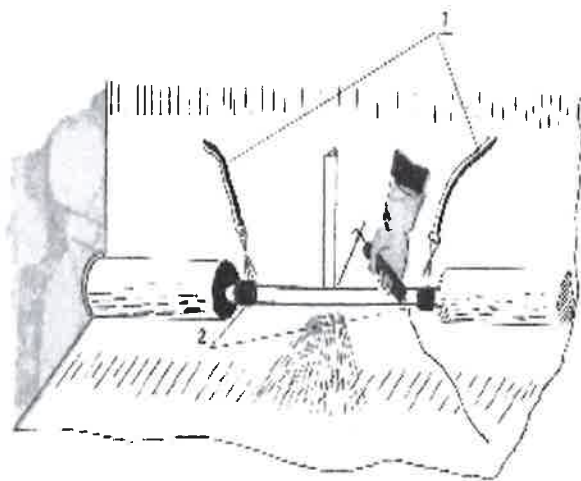
Rys. 3. Z izolowanych rurociągów, na których prowadzi się prace spawalnicze, należy usunąć izolację cieplną na odcinku gwarantującym bezpieczeństwo, a w razie potrzeby chłodzić skutecznie: 1- przewody doprowadzające wodę, 2- zwoje mokrej tkaniny.
