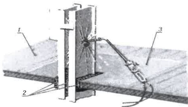
Rys. 4. Elementy instalacji, rozgrzewające się przy spawaniu od płomienia lub na skutek przewodnictwa ciepłego, stykające się z materiałami palnymi należy zdemontować lub skutecznie chłodzić: 1- palna ścianka, 2- niepalna wykładzina, 3- haki podtrzymujące instalację.
